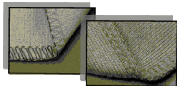
Figura 4. Puntadas 504 y 514 de Sobrehilado / Ribeteado.
